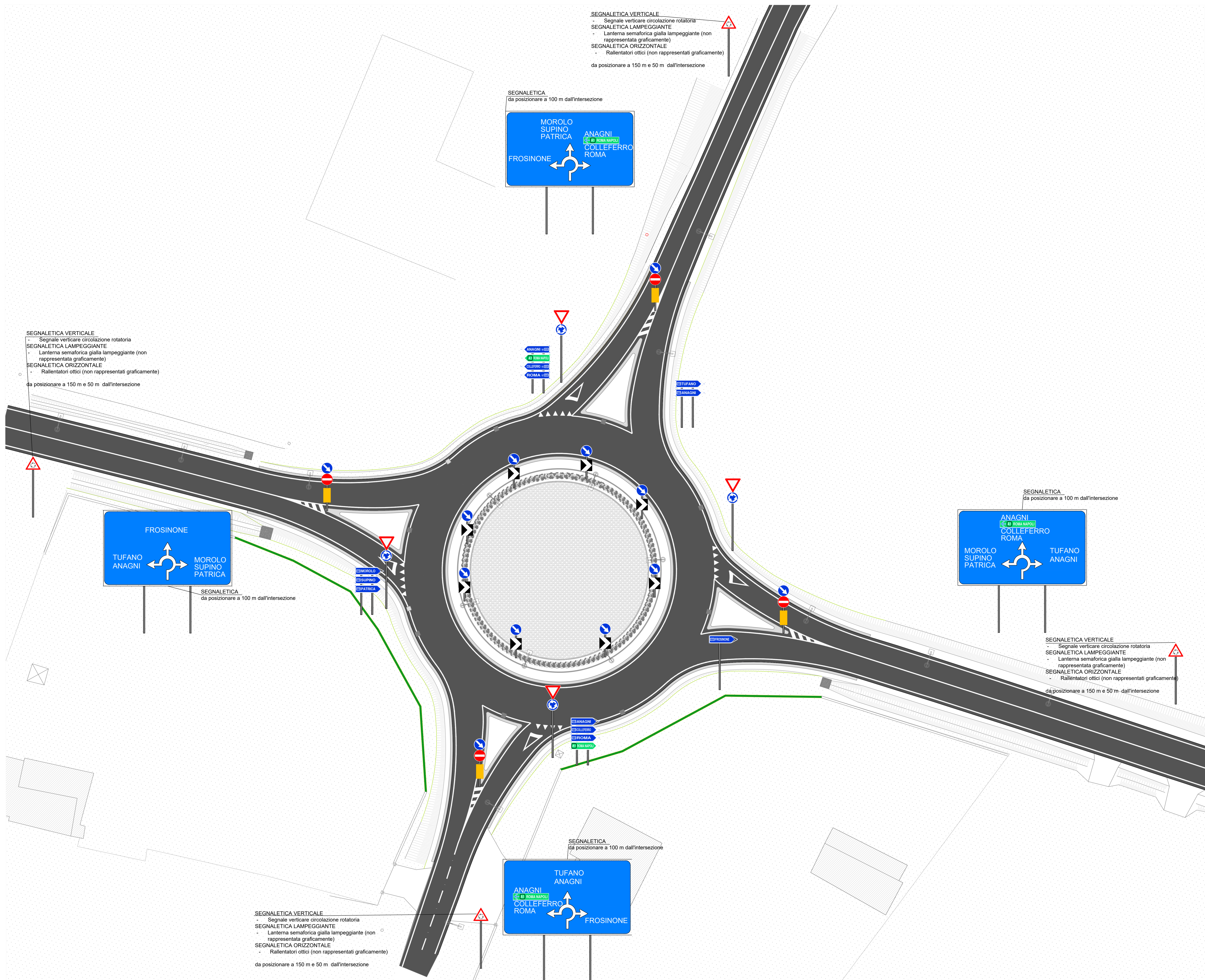
PLANIMETRIA SEGNALETICA ORIZZONTALE E VERTICALE scala 1:200
